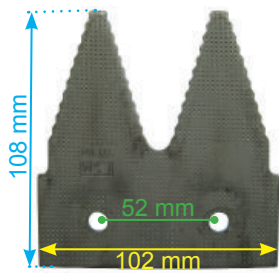
153-3211041, Bjelkeblad dobbelt
