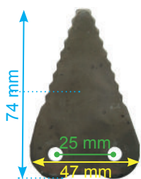
153-3211221, Bjelkeblad enkelt
